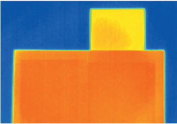
РИС. 10. ◀ Изображение, полученное при помощи ToF-камеры. Объекты одинаковой высоты выглядят как единый объект
