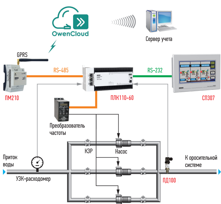
РИС. 1. ► Функциональная схема управления насосной станцией
