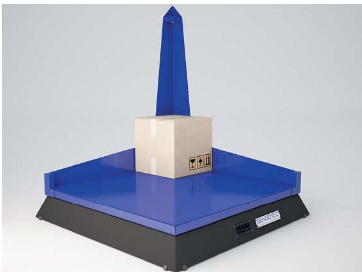
РИС. 1. Система SENSOTEC Volume One
