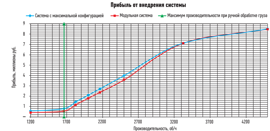
РИС. 3. ▼ Прибыль от внедрения модульной системы и системы с максимальной конфигурацией
