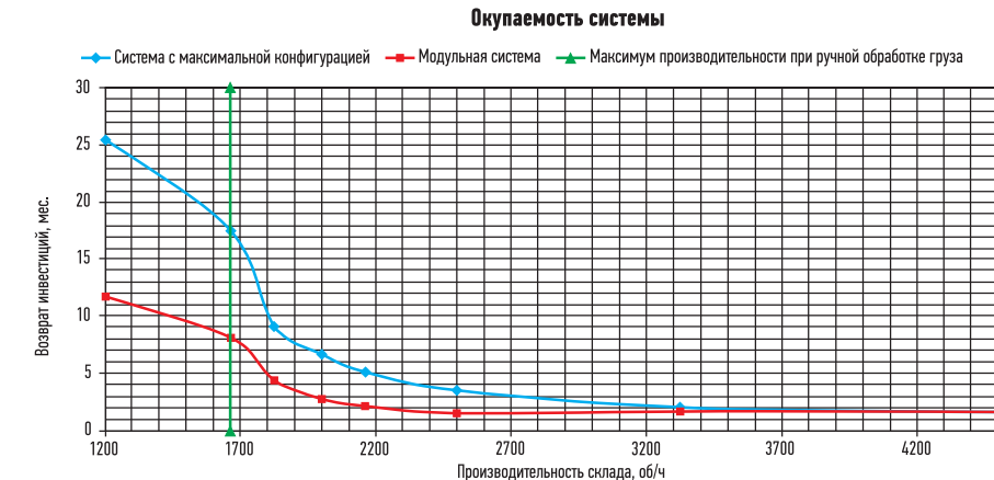
РИС. 2. ▲ График возврата инвестиций при использовании модульной системы и системы, спроектированной под увеличение производительности в 2,5 раза
