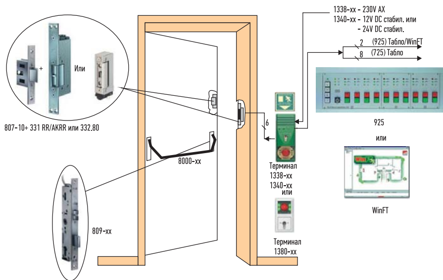
РИС. 2. ▲ Система effeff для эвакуационных и аварийных выходов
