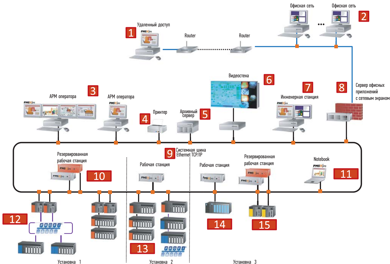
РИС. 1. ▼ Архитектура PCSU PMSXpro
