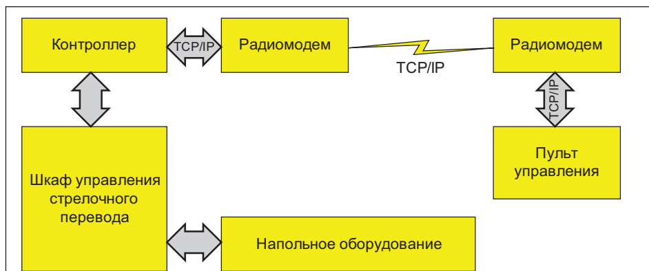
Рис. 1. Структурная схема дистанционного контроля и управления стрелочным переводом
