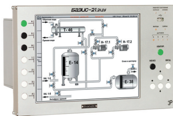
Рис. 10. ▶ Исполнение БАЗИС-21.2ЦУ
