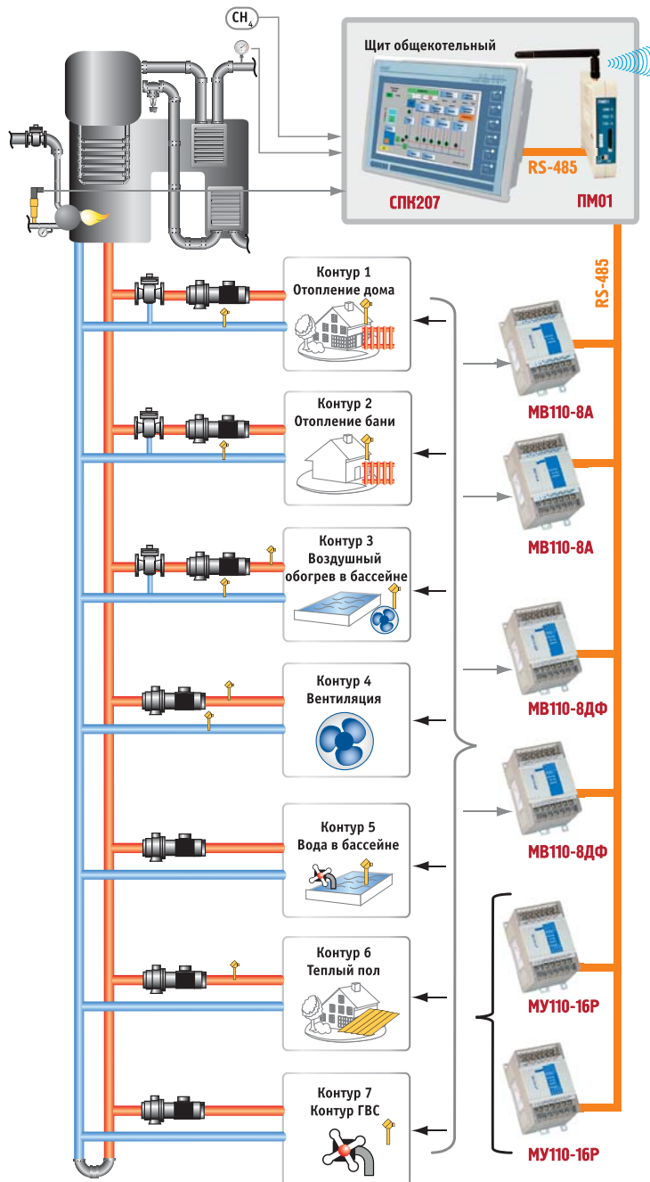
РИС. 1. ◀ Функциональная схема управления
